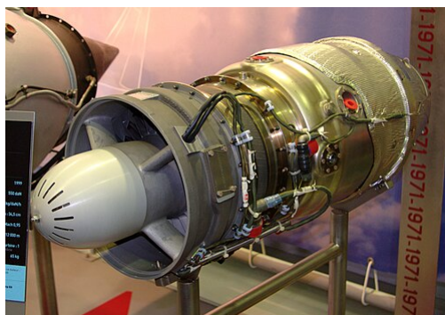
Турбореактивный двигатель Microturbo TRI 60-30, используемый на Storm Shadow, Аэрокосмический музей Сафран
